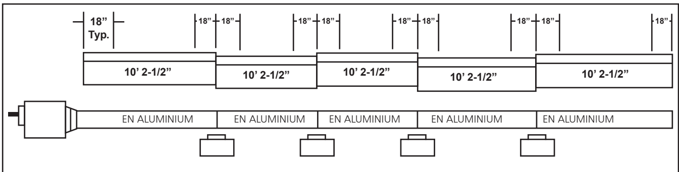
FIGURE 2G : Modèle Ener-Radiant Ener-Radiant XL Model ERXL-150, ERXL-175
