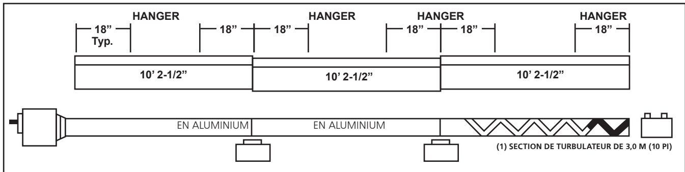
FIGURE 2D : Modèle Ener-Radiant Ener-Radiant XL Model ERXL-100
