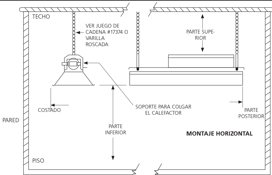
Figura 4. Distancias a combustibles
